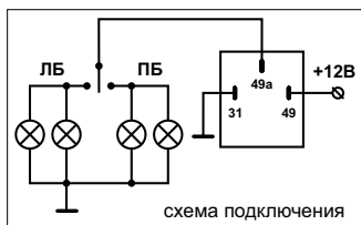
схема подключения
